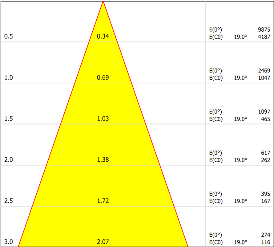
Расстояние [m] Диаметр конуса [m] C0 - C180 (Полу-угол: 38.0°)
